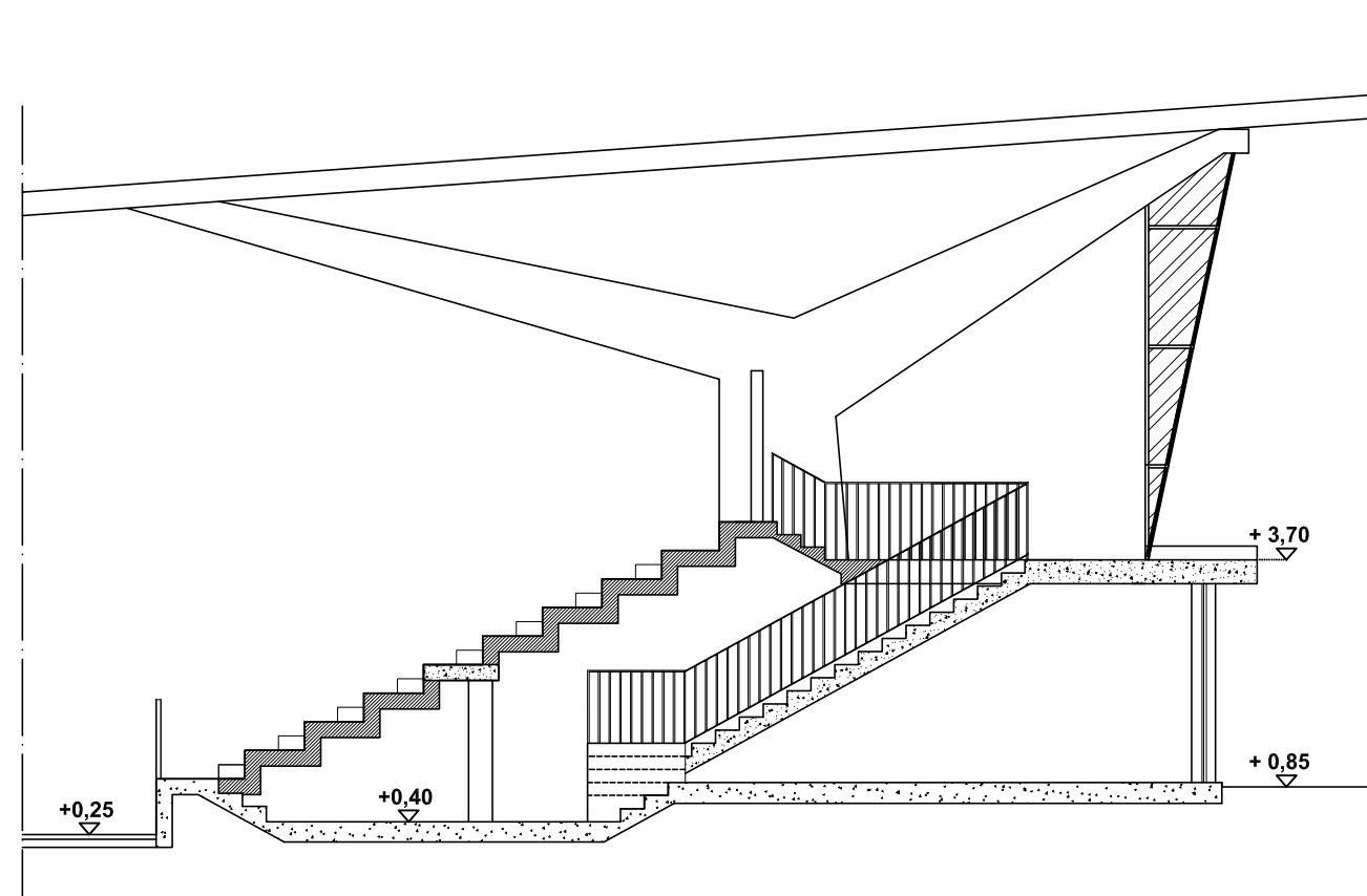
SEZIONE A-A - Scala 1:100
